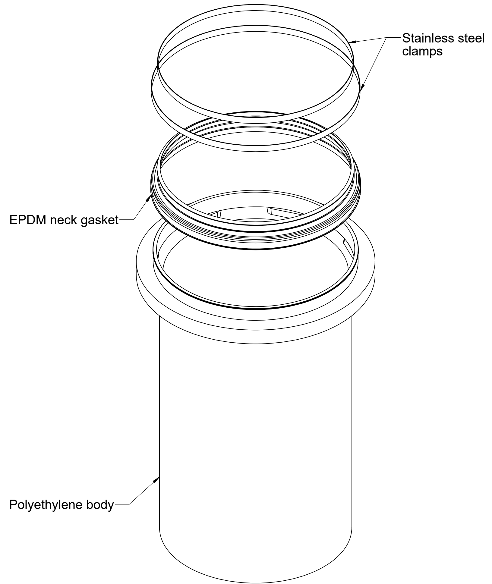
LONG RISER (LR-24)
