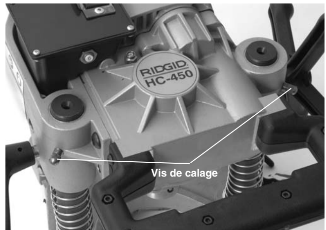
Figure 13 – Réglage des vis de calage
