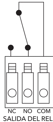
Relé activo/encendido
