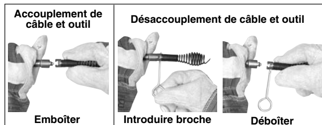
Figure 10 – Accouplement et désaccouplement des outils
