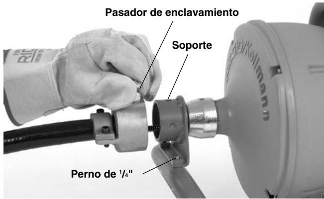
Figura 4 – Montaje de la manguera guía a la nariz de la K-40
