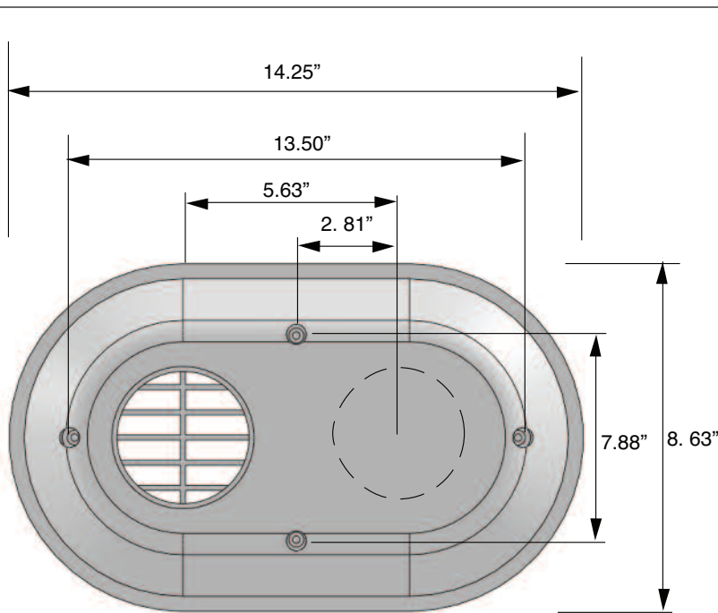
Fig. 3: Vent Termination Dimensions
