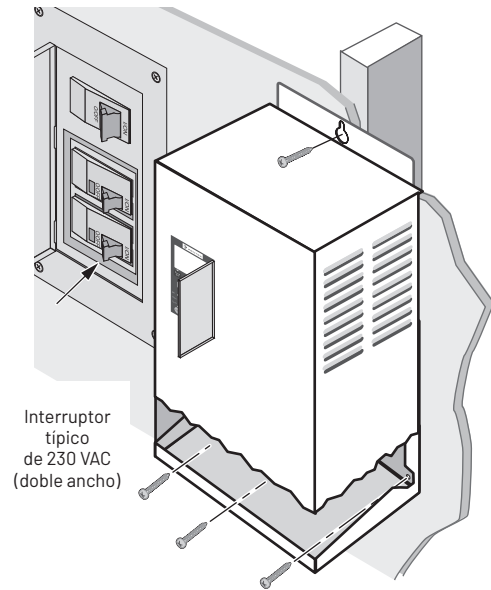
Figura 6 - Separe la tapa de la placa trasera
