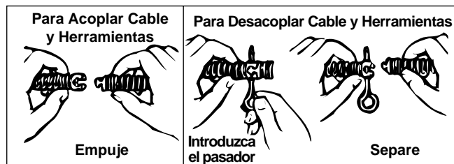
Figura 6 – El acoplamiento y desacoplamiento de herramientas
