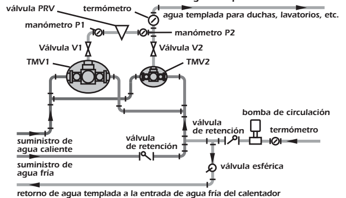
Diagrama 3 Instalación de sistema HI-LOW remoto con recirculación de agua templada
