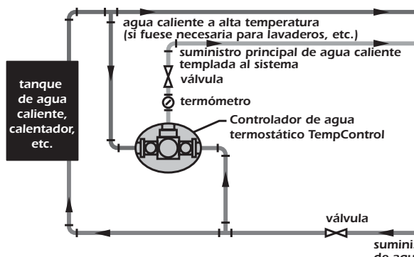
Diagrama 1 Instalación de una sola válvula en o cerca de la fuente de agua caliente
