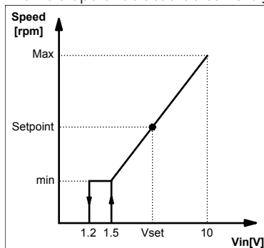
Cifra 6: Entrada de voltaje detectada
